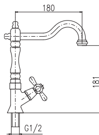
MK194/8 MK594/8 Chrom – Chrome – Хром
